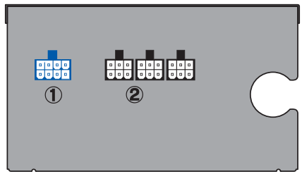
①PCI-EXPRESS コネクタケーブル用 ②Serial ATA & FDD & Driver コネクタケーブル用
